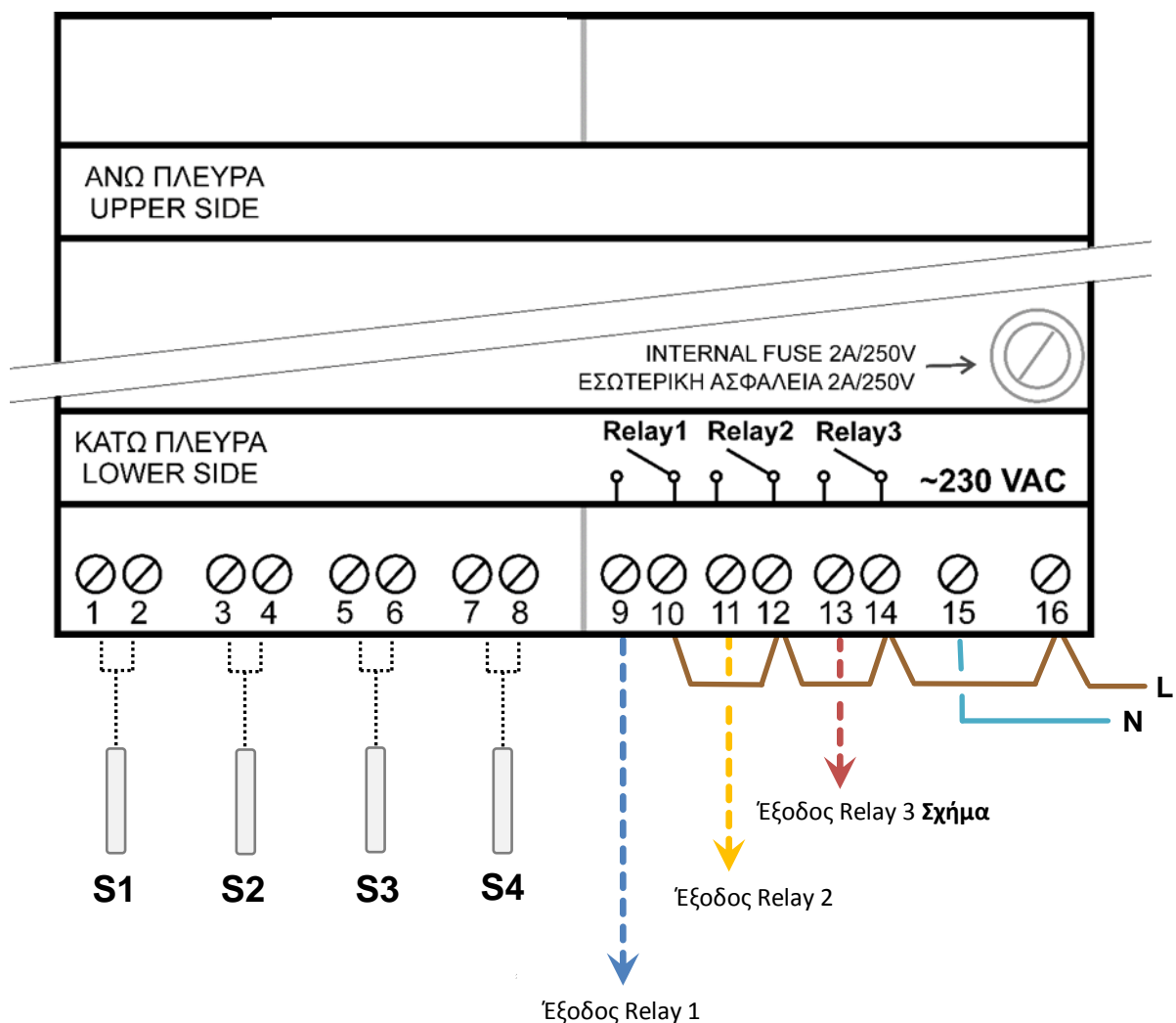
Σχημα 1- Σχέδιο εγκατάστασης
